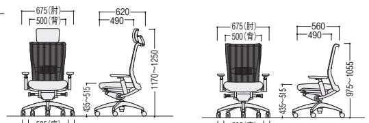
TS-5775・5755
